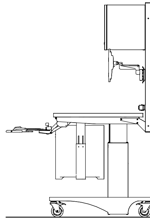
Elevation B
