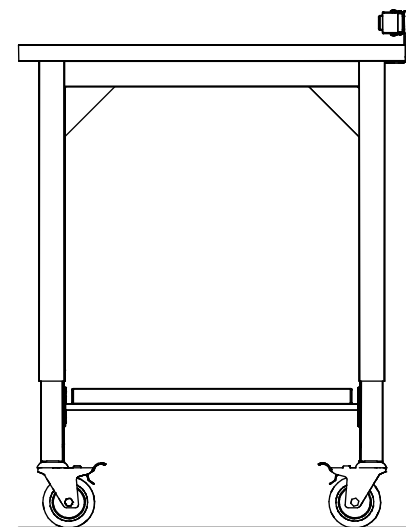
Elevation B
