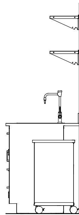
Elevation B
