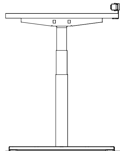
Elevation B
