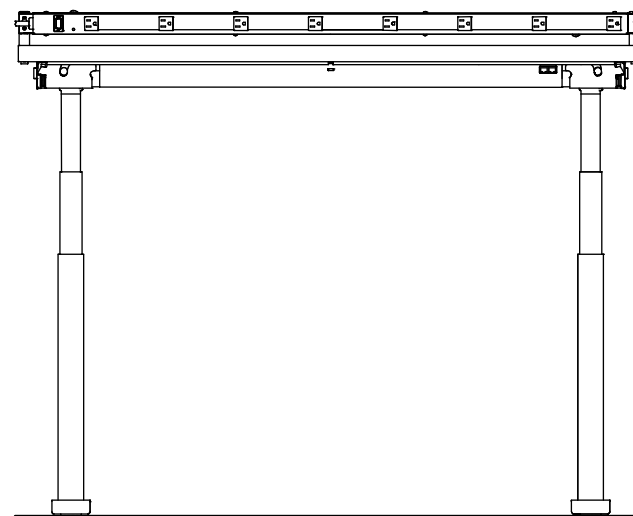
Elevation A
